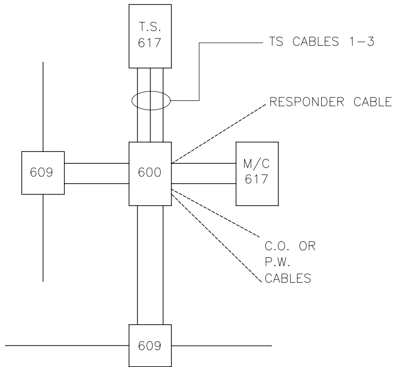
MINI CARRIER TS SITE LAYOUT
